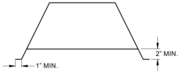
END ELEVATION
