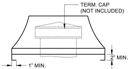
END ELEVATION
