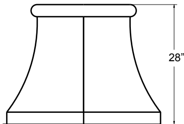
END ELEVATION
